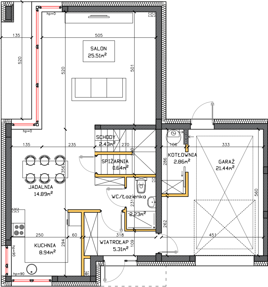
RZUT PARTERU
