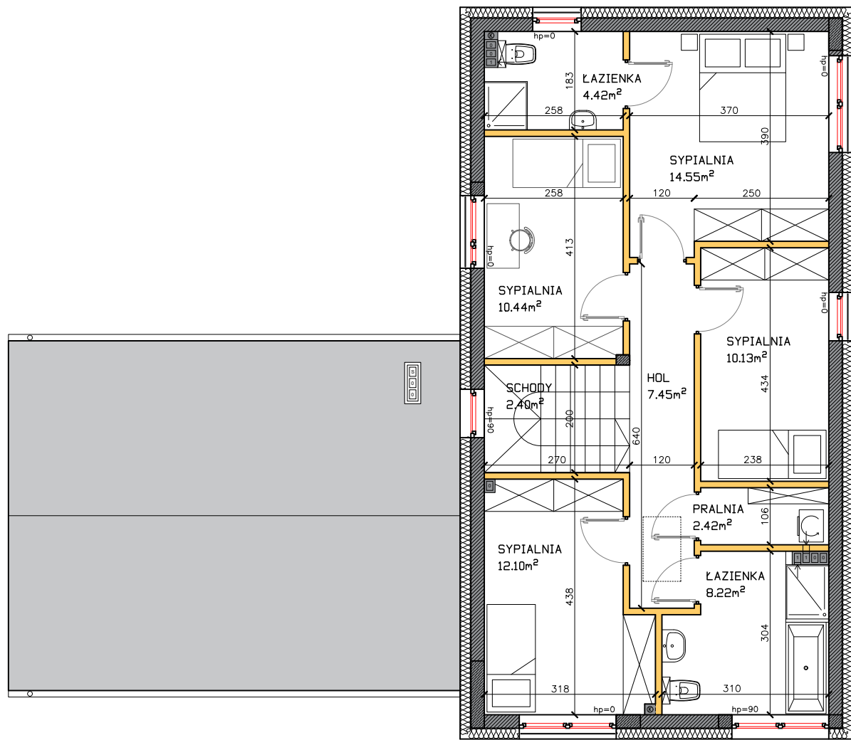
RZUT PIĘTRA
