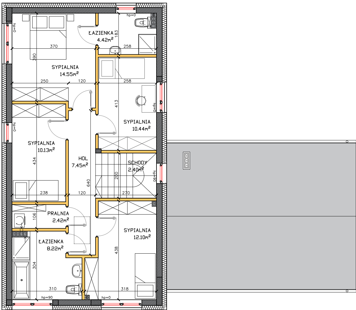
RZUT PIĘTRA
