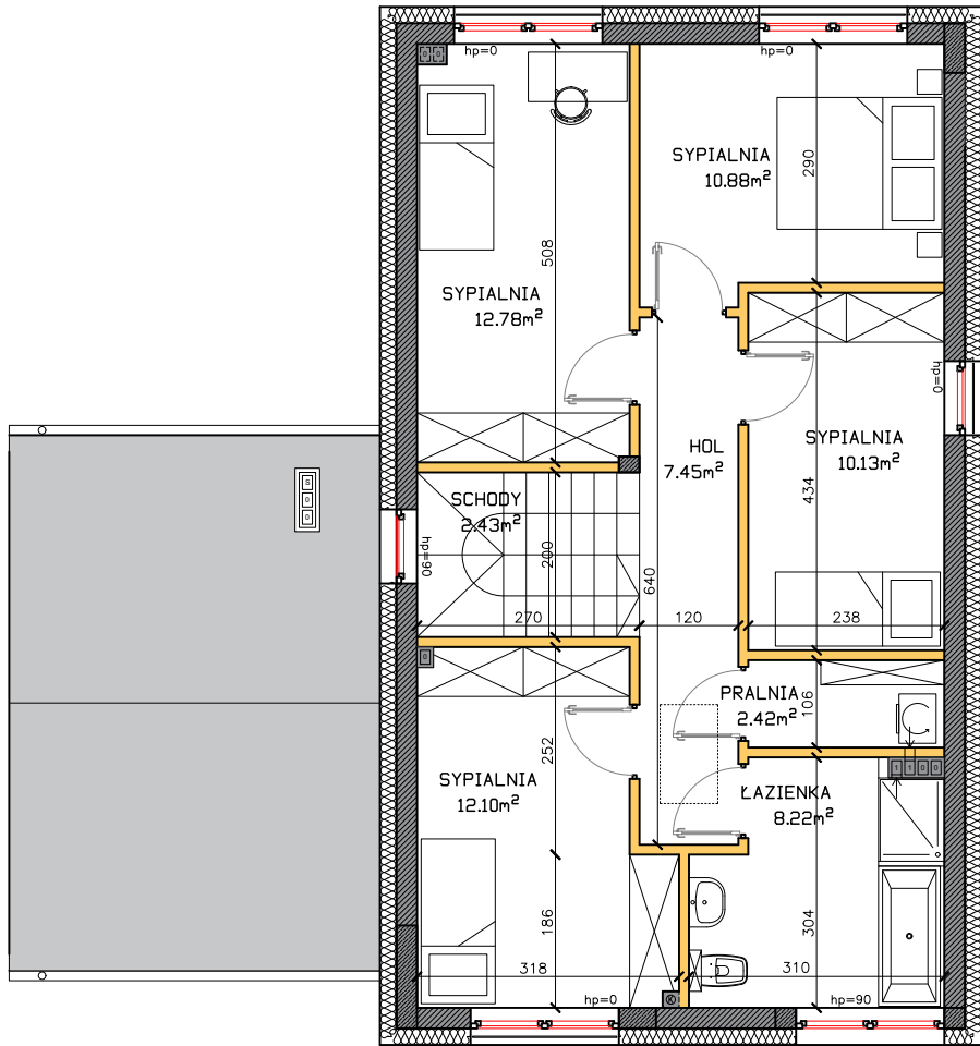
RZUT PIĘTRA
