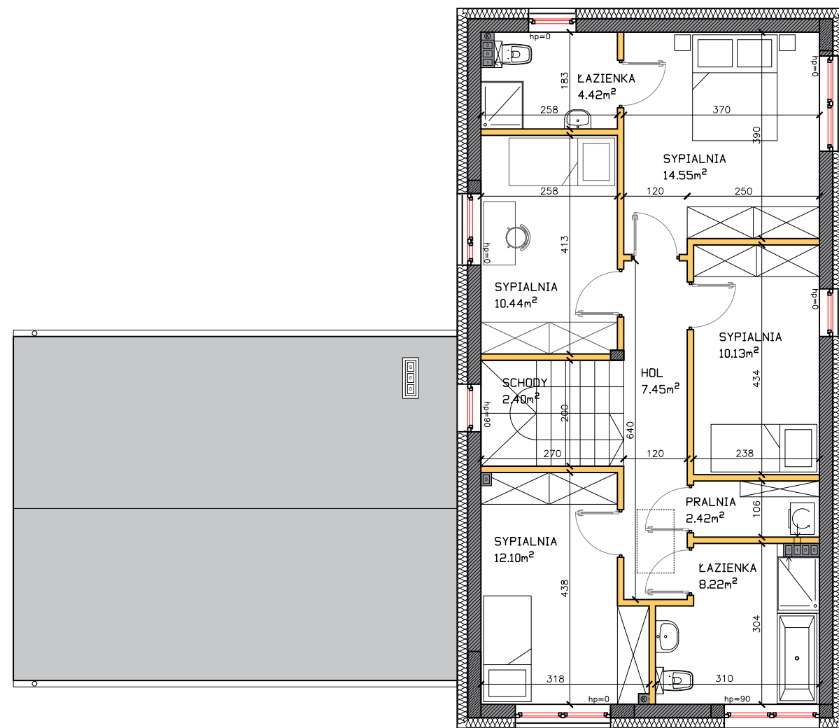
RZUT PIĘTRA
