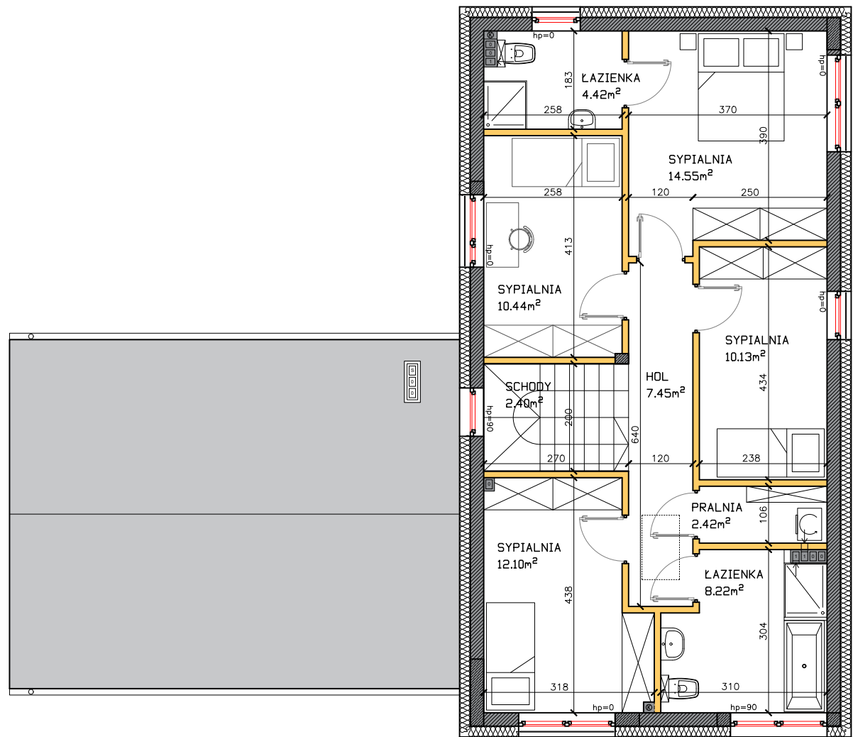
RZUT PIĘTRA
